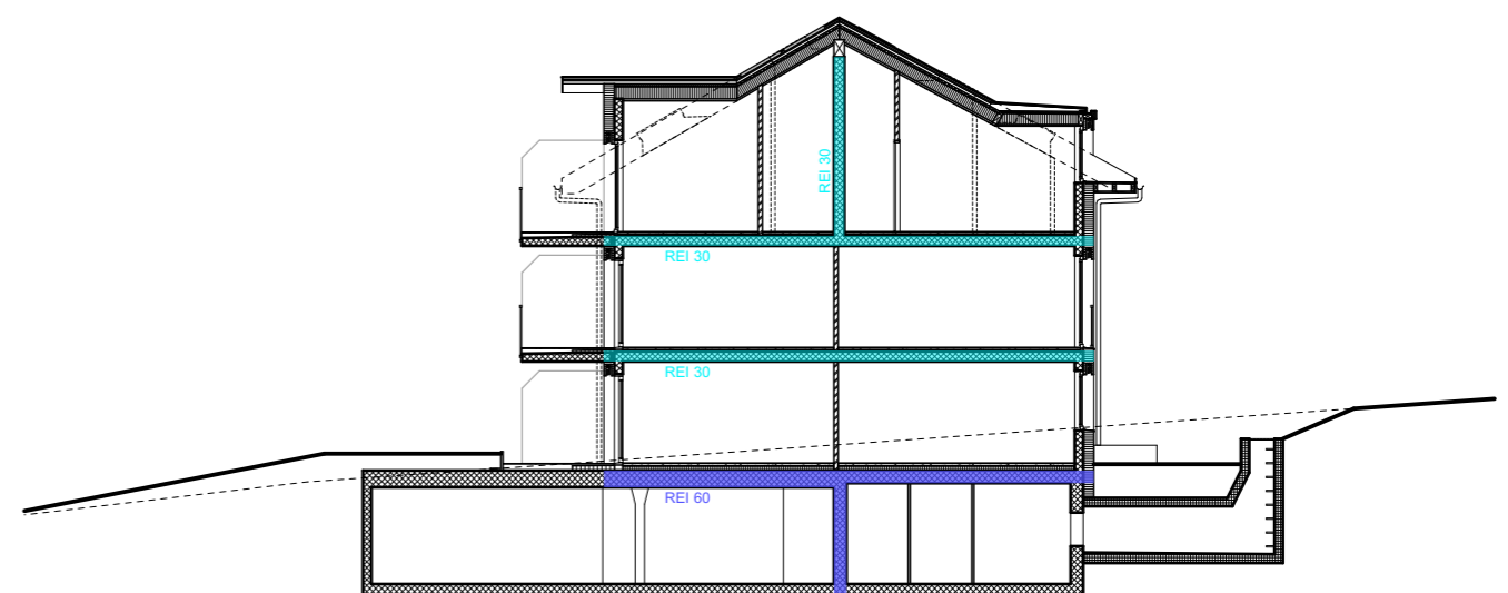
COUPE A-A
