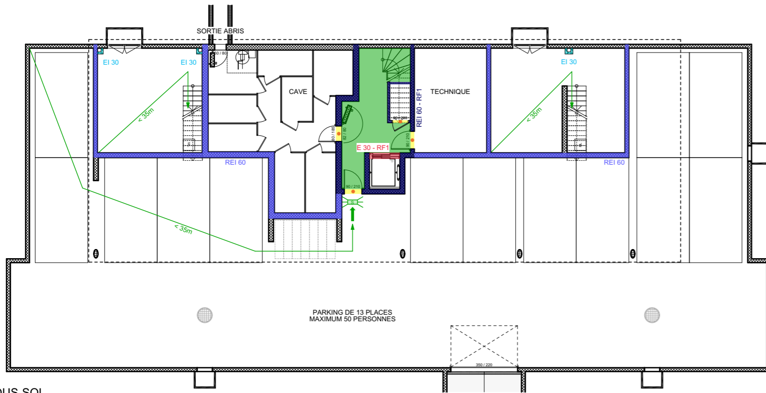
SOUS-SOL
