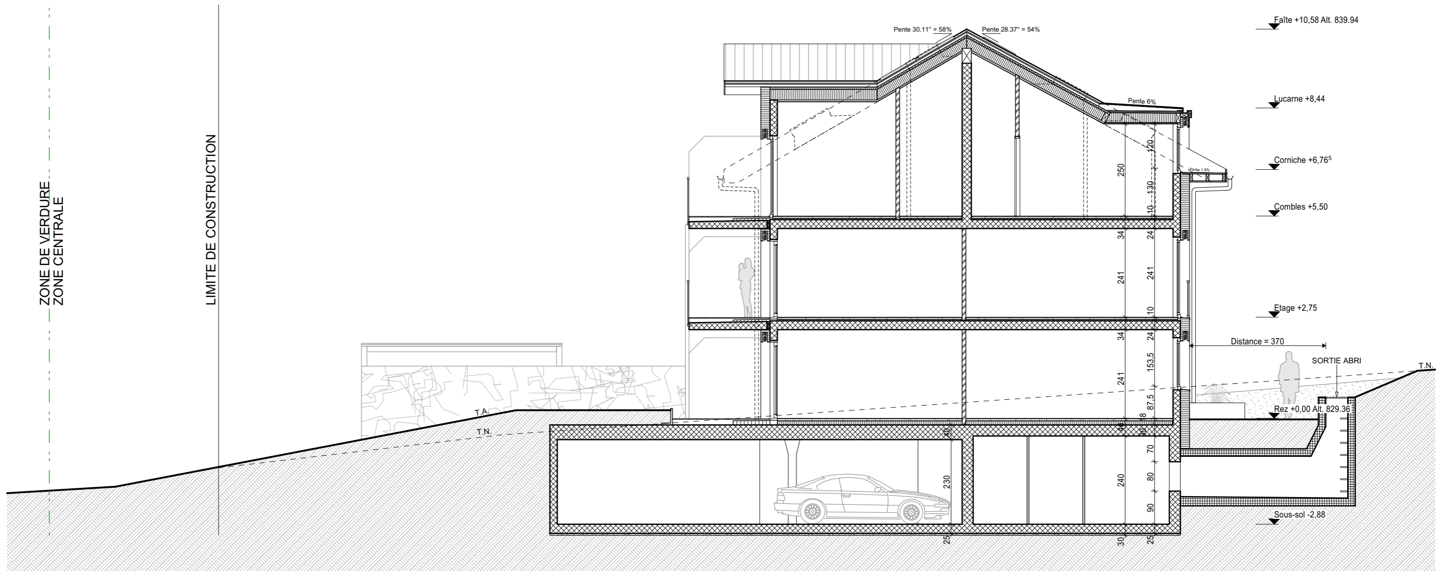
COUPE A-A
