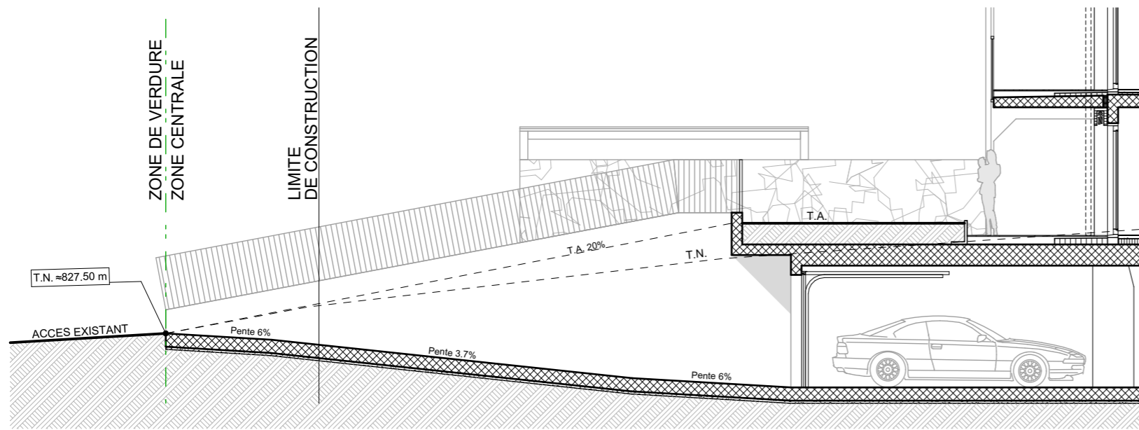
COUPE A'-A' - SUR LA RAMPE DE PARKING
